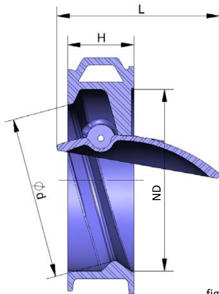
A-A SECTION
